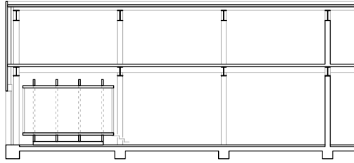
Schnitt 1:300
