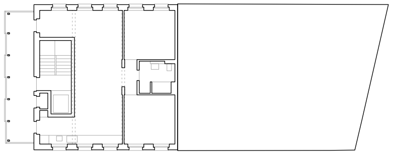
1. Obergeschoss 1:300
